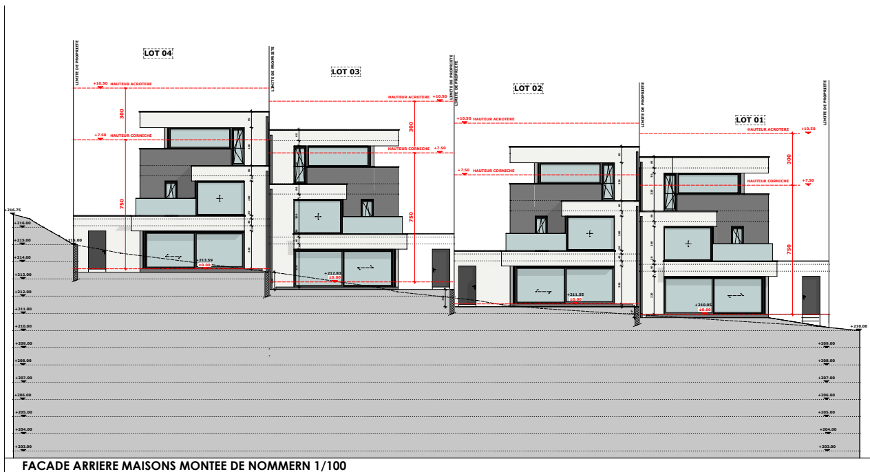
FACADE ARRIERE MAISONS MONTEE DE NOMMERN 1/100
